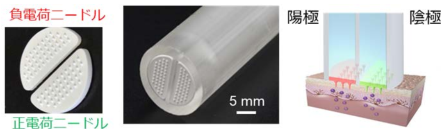
図 1 デュアルニードルポンプの構造とイオントフォレーシスへの応用
